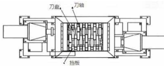
图6 撕碎机俯视结构图
