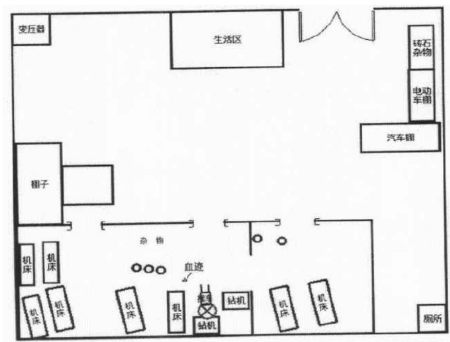
(图1 事故现场方位示意图)
