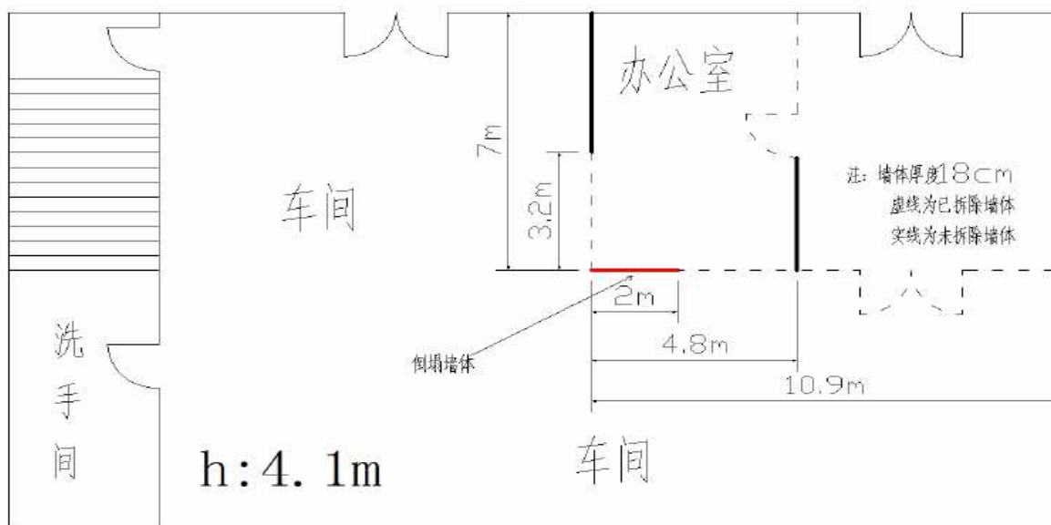
图 4 隔墙拆除平面图
