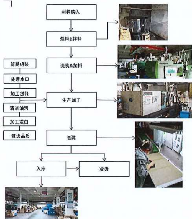
图2 东恒公司塑胶制品生产流程图
