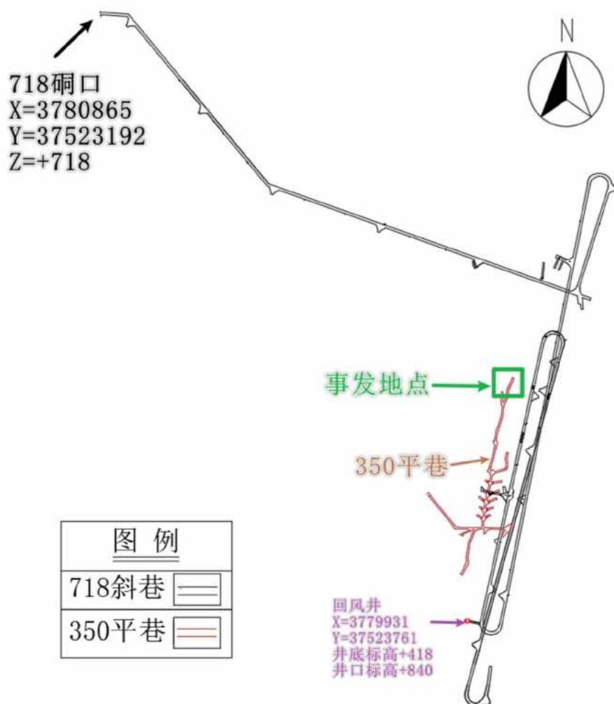
图 2 PD718 井巷工程示意图
