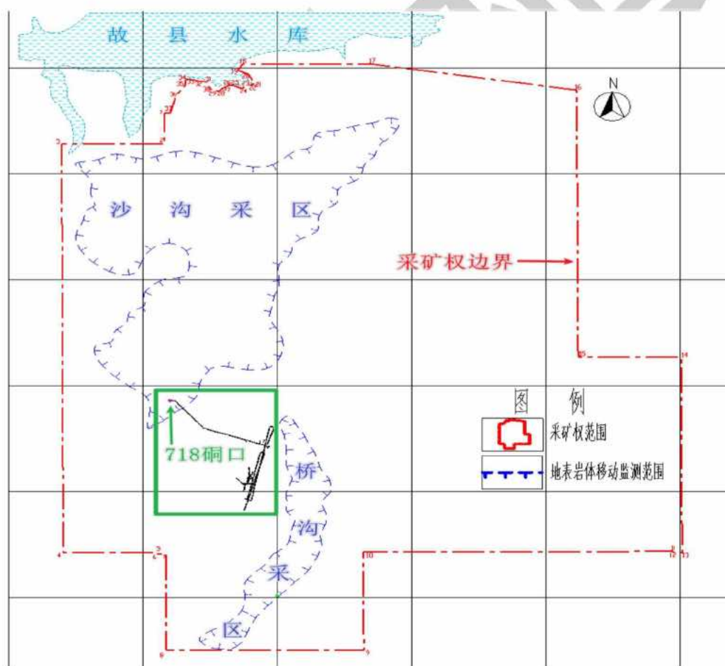
图 1 矿区采区设置情况及 PD718 硐口位置示意图
