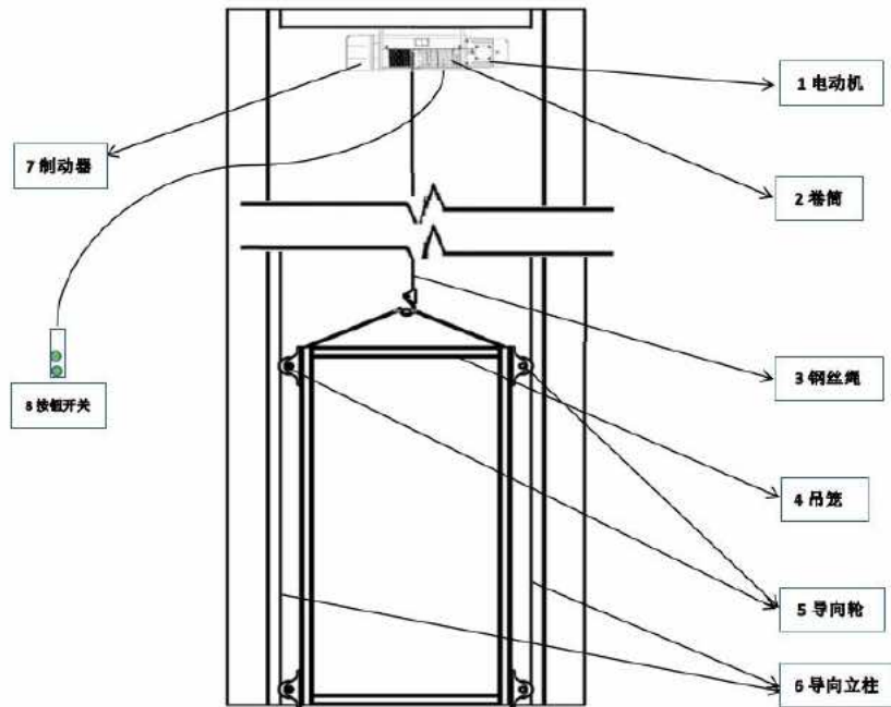
图4 涉事设备构成示意图
