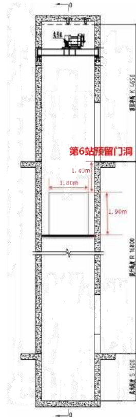
图4 电梯井道
