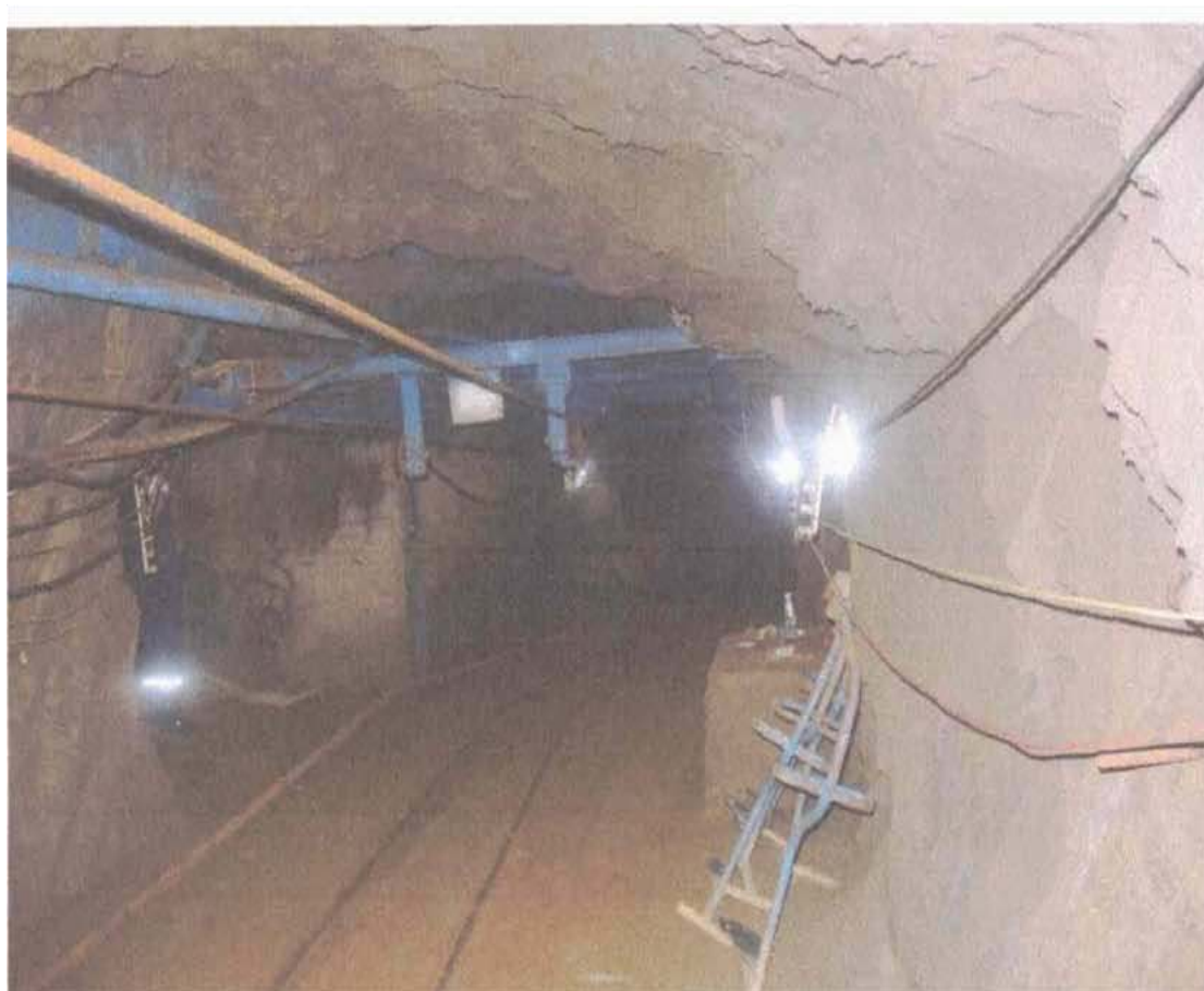
（图示 1）图片说明：大源探矿点-180 中段车场
