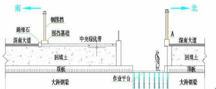
围挡基础支撑支架拆除后状态
