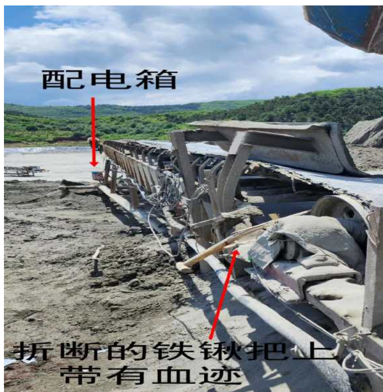
图3 11号带式输送机北侧
