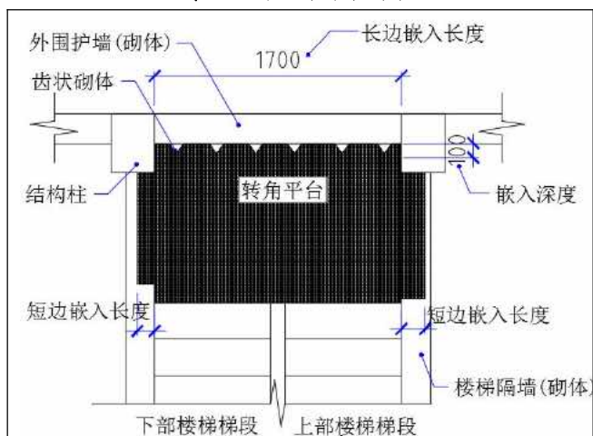
图 11 拆除前转角平台嵌固支座平面示意图 (mm)
