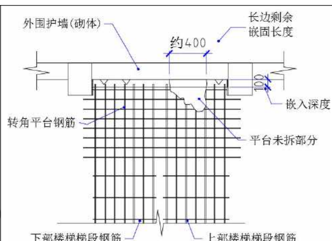
图 12 坍塌前转角平台平面示意图 (mm)
