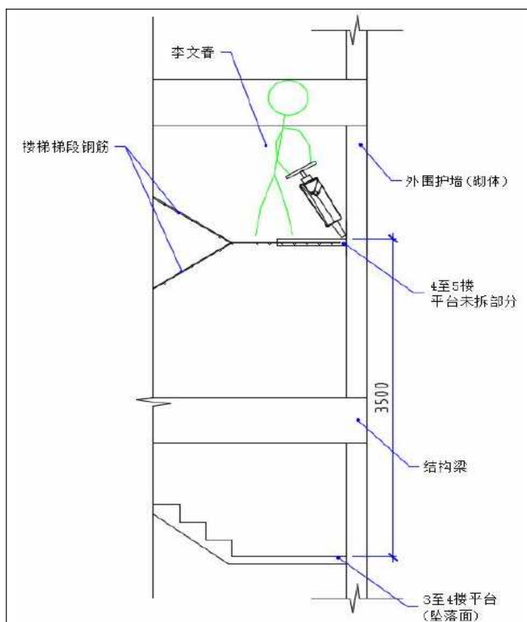
图 13 坍塌前事故楼梯拆除工况示意图(mm)
