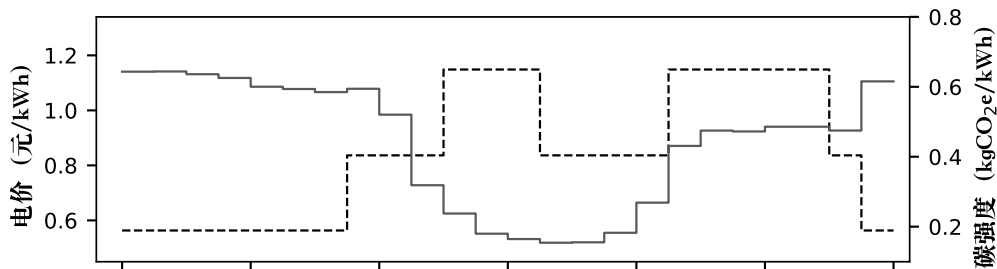
(a) 分时电价与时变碳强度输入
