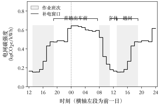
(a) 电网碳强度与补电窗口
