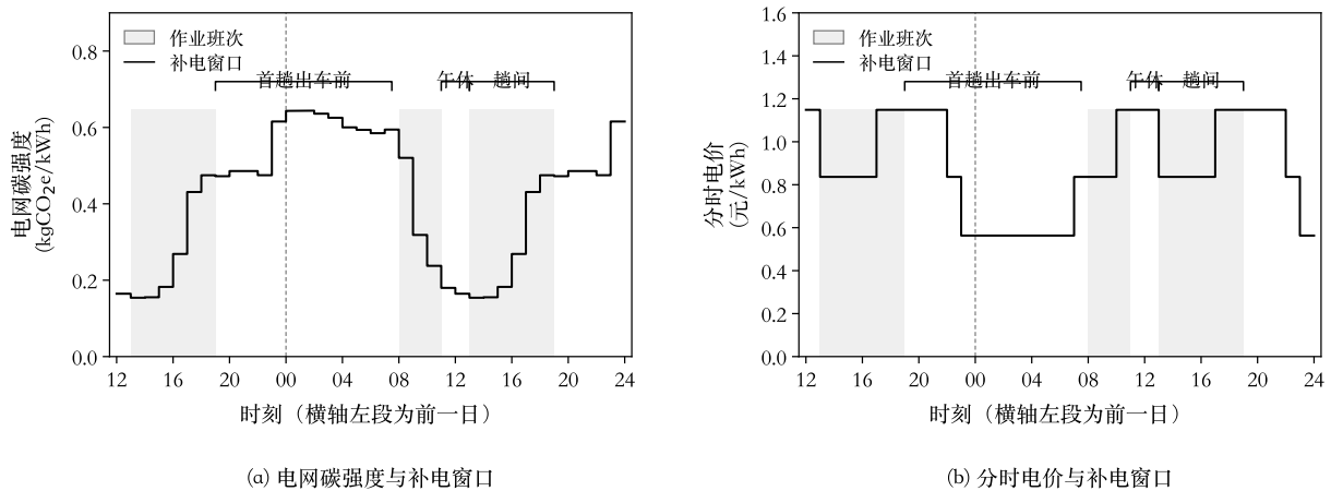
图4 分时电价、电网碳强度与可充电时段的对应关系 (横轴左段表示前一日)
