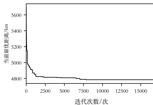
图 3 本文算法在 PR17B 上的收敛过程
