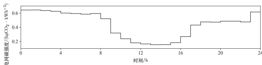
图 2 TVGCI-CMDMF-DVRP 算例的逐时电网碳强度
