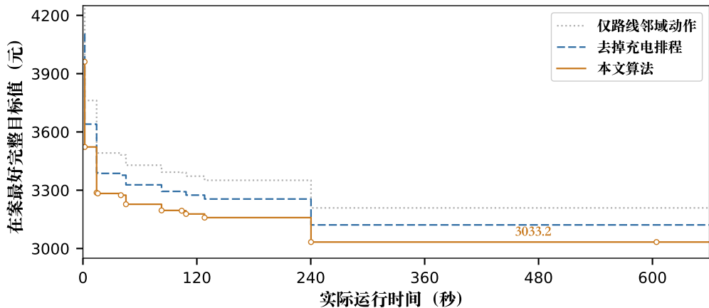
三条消融臂在同一预算下的收敛过程
