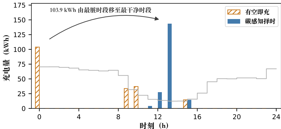
(b) 同样充 189.3 kWh，两种规则把它放在完全不同的时刻
