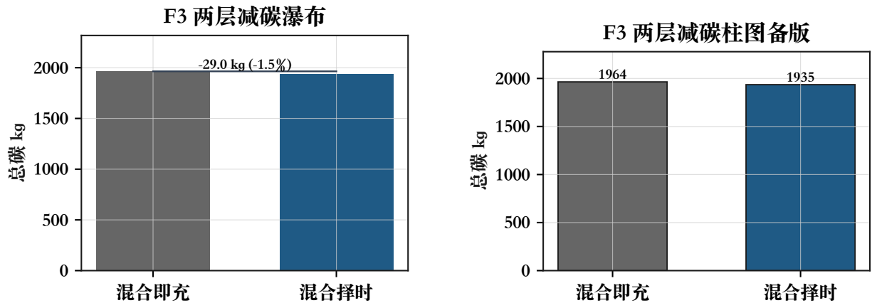
图 3 两层减碳效果
