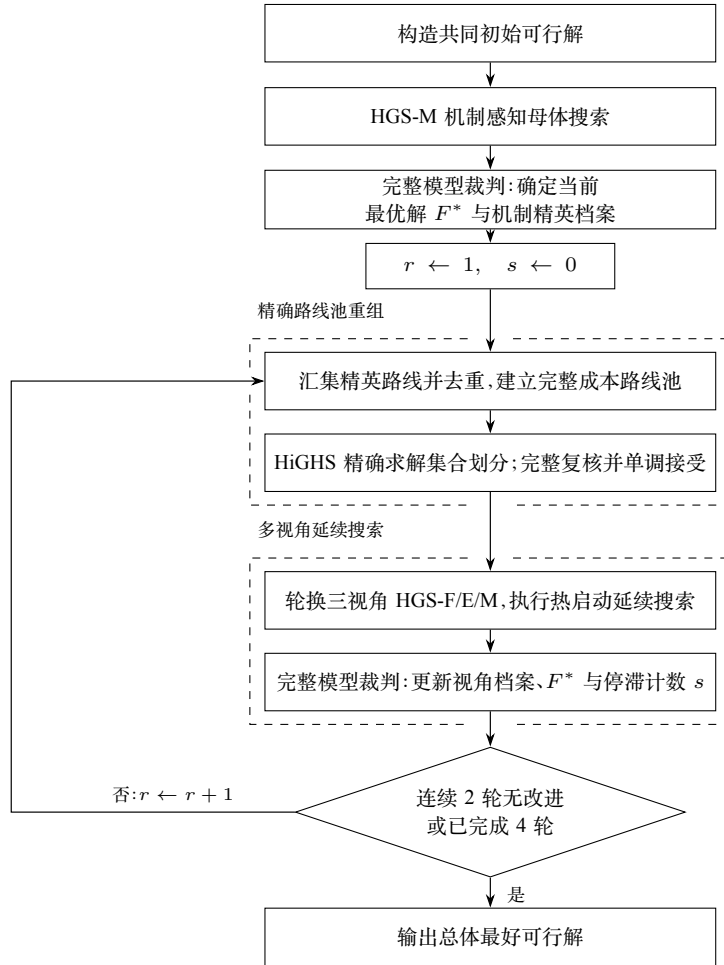
图1 MV-HGS-SP 算法主流程
