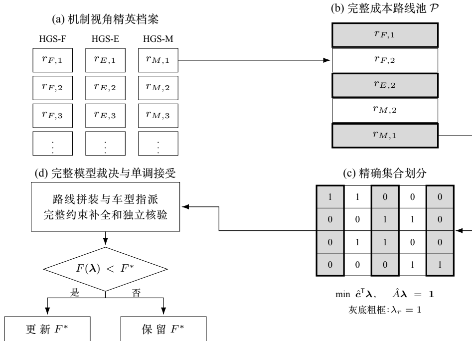
图2 三视角路线池与集合划分重组示意
