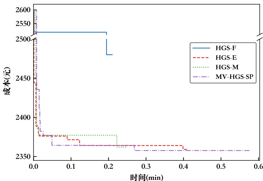
图4 不同算法迭代图
