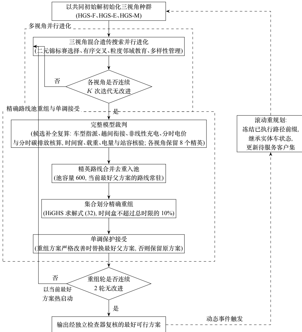
图1 MV-HGS-SP 算法流程
