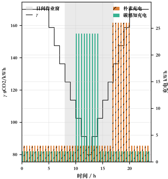
(a) 电网碳强度与30分钟充电负荷
