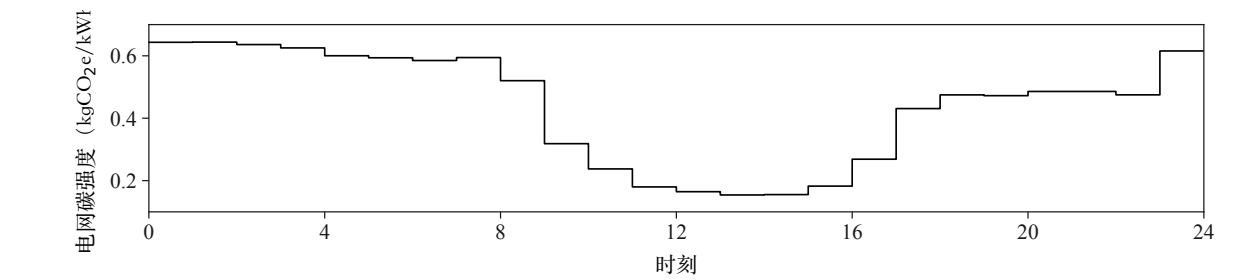
图 2 TVGCI-CMDMF-DVRP 算例的逐时电网碳强度
