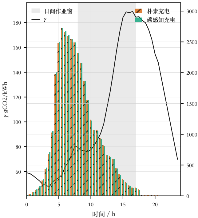
(a) 48槽碳强度与充电负荷
