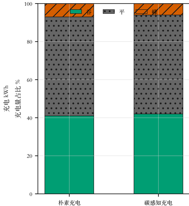
(b) 峰/平/谷充电占比
