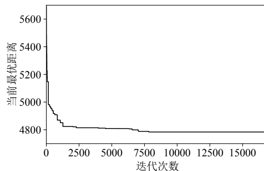
图 4 本文算法在 PR17B 上的收敛过程
