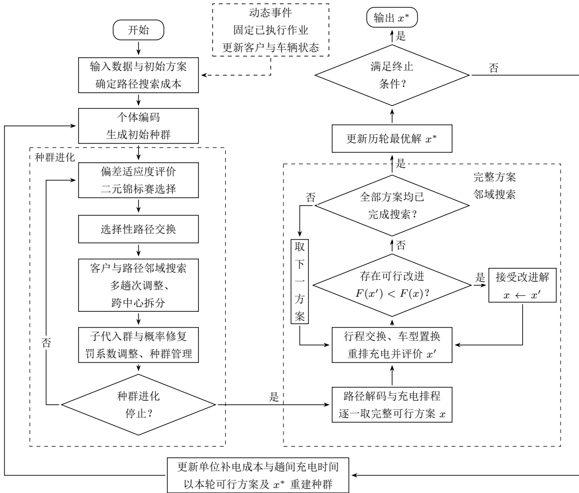
图 1 MTC-HGS 算法流程图
