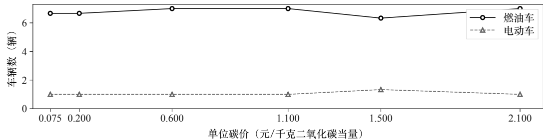
图 4 不同碳价下的车辆派遣数量
