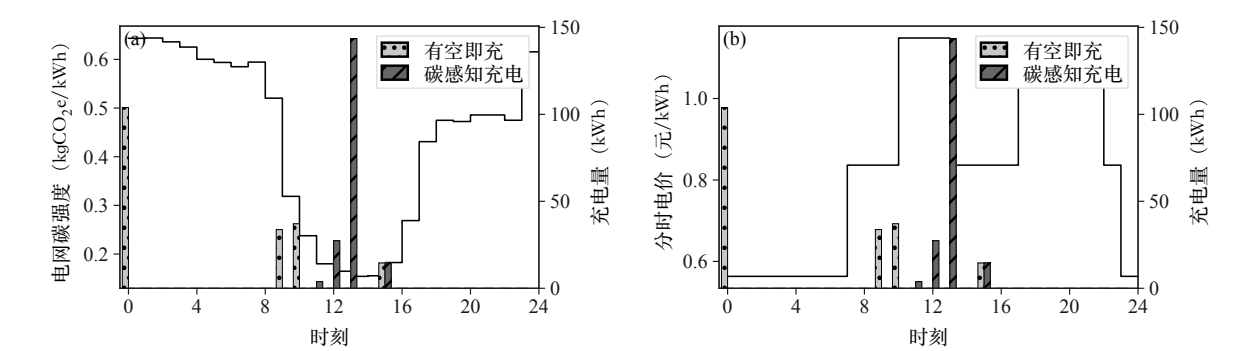
图 5 分时电价、电网碳强度与车辆充电时刻
