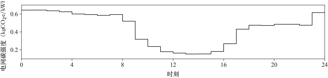
图 2 北京代表日电网碳强度时变曲线
