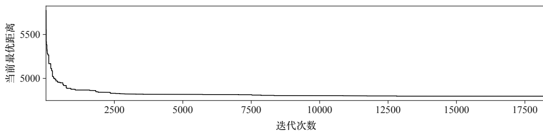
图 3 本文算法在 PR17B 上的收敛过程
