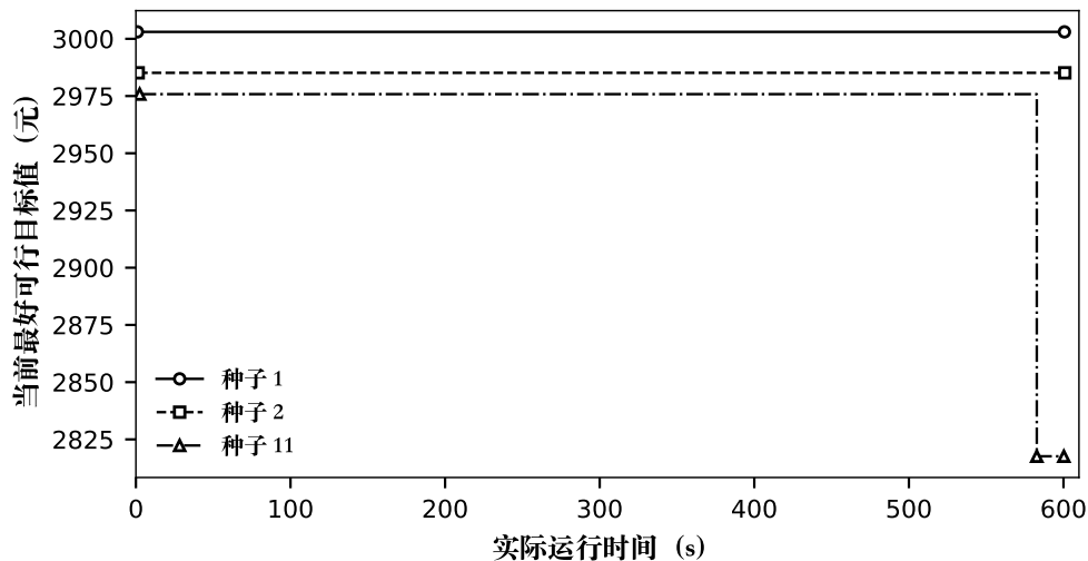
图2 本文算法在仿真实验中的收敛过程
