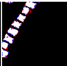
ChangeMamba-B
