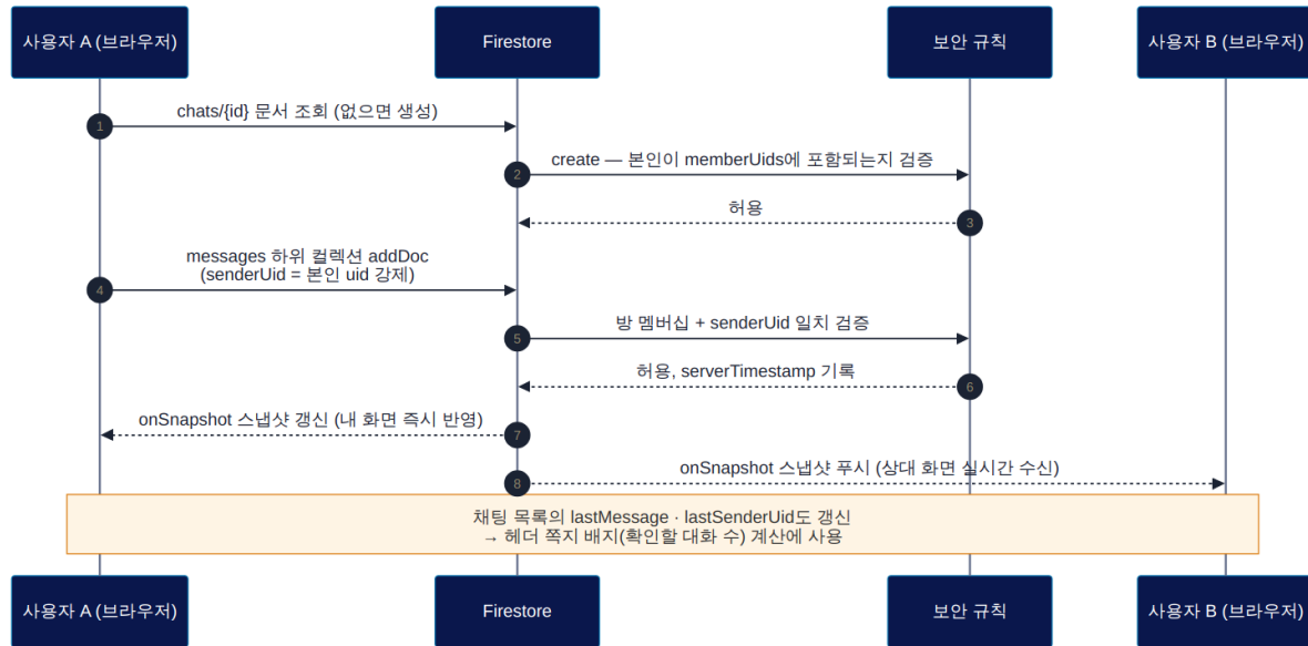
[SF-02] 실시간 채팅 메시지 송수신 시퀀스
