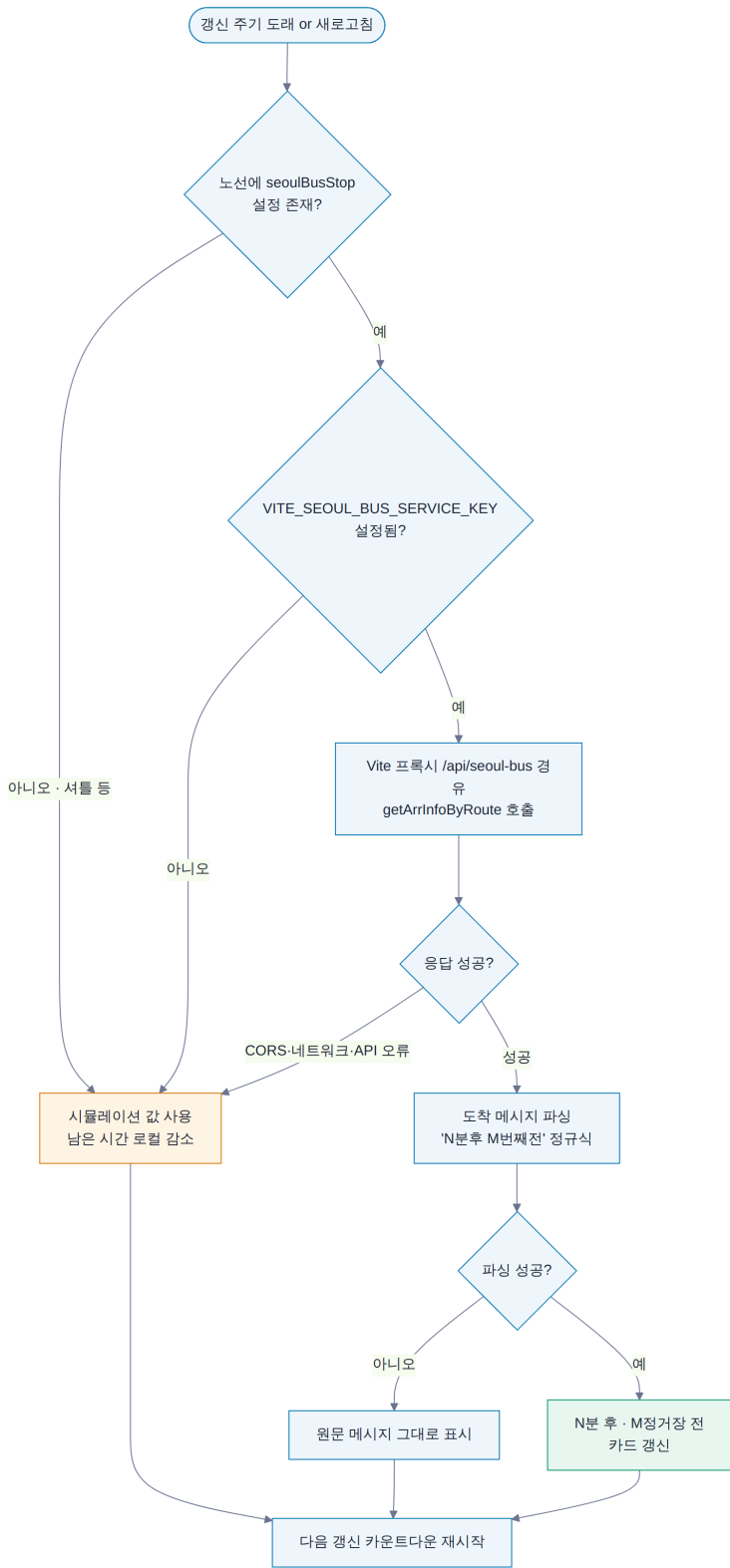
[SF-03] 버스 실시간 도착정보 조회, 폴백 흐름
