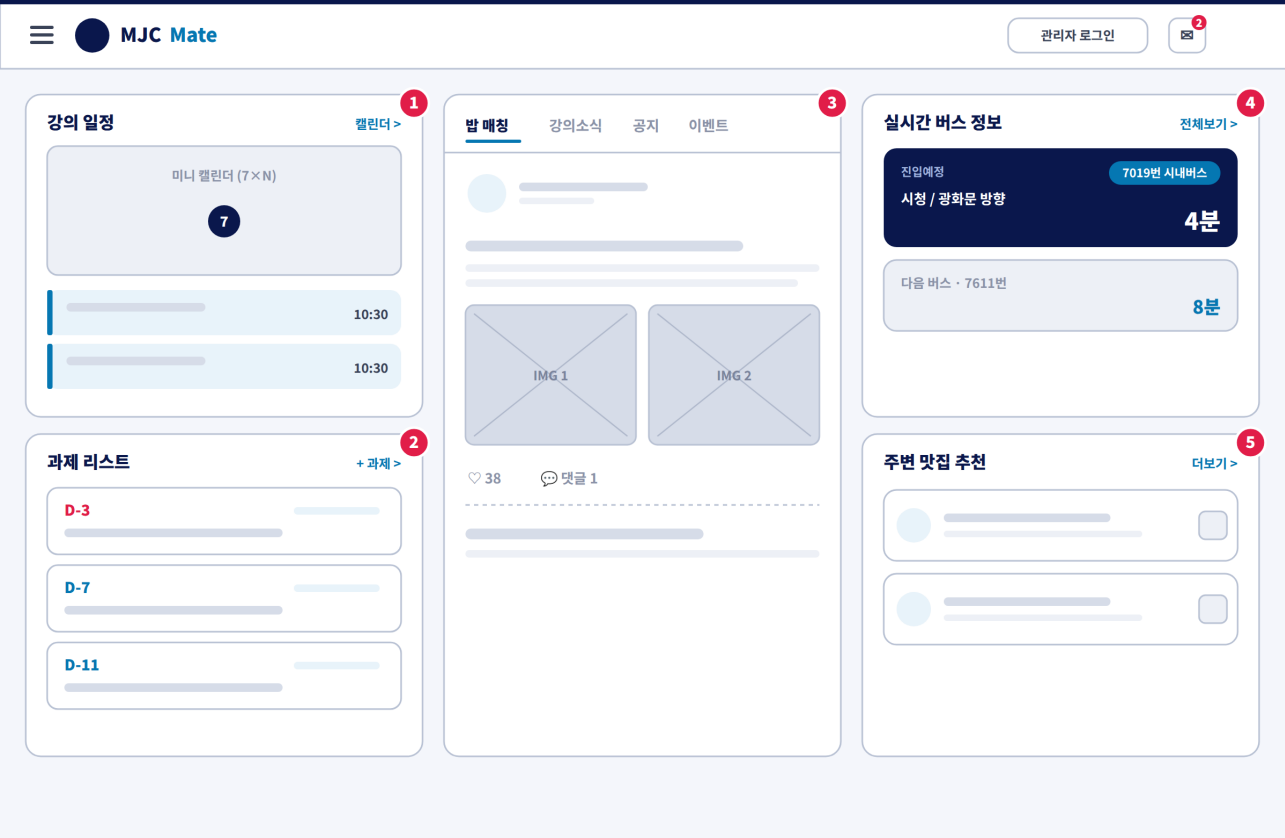
[SCR-01] 홈 대시보드 — 와이어프레임 (번호는 아래 구성요소 표와 대응)
