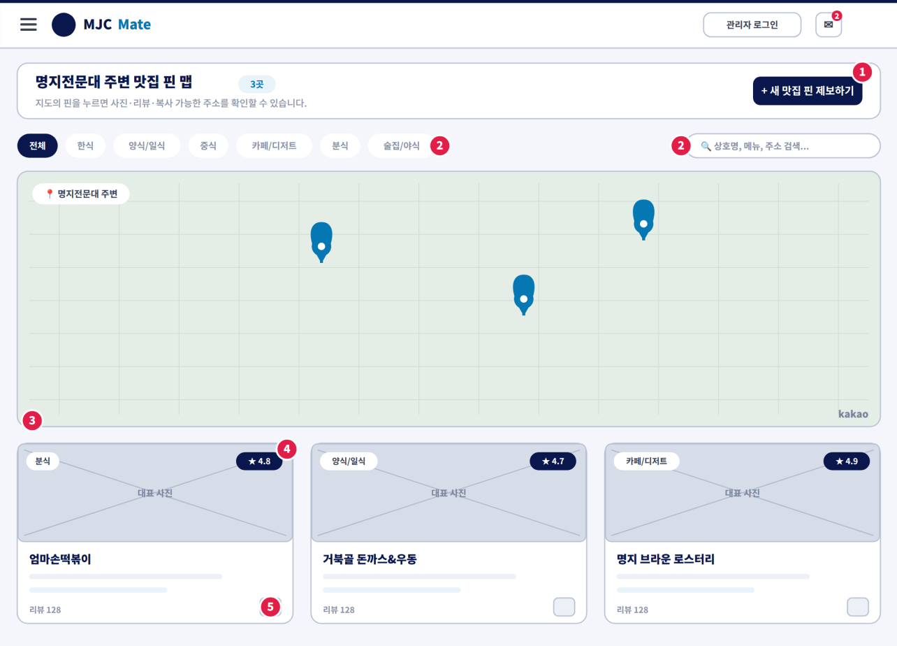
[SCR-03] 주변맛집 (카카오맵) — 와이어프레임 (번호는 아래 구성요소 표와 대응)
