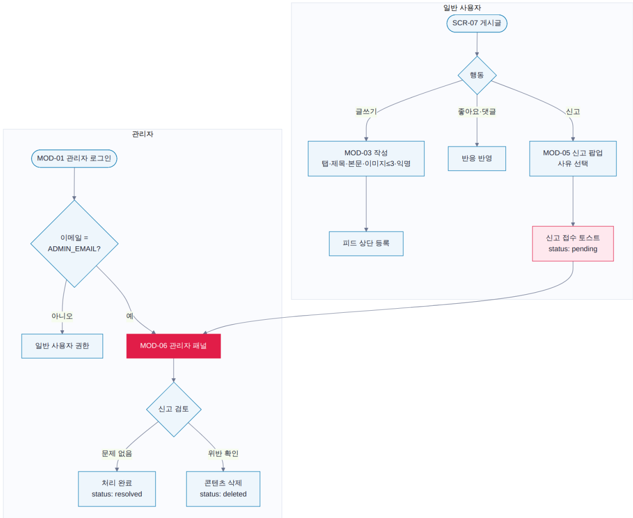
[UF-04] 게시물 작성 · 신고 → 관리자 처리 플로우
