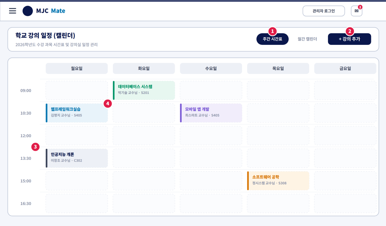
[SCR-04] 강의일정 — 와이어프레임 (번호는 아래 구성요소 표와 대응)
