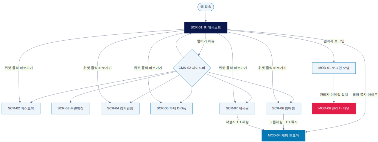
[UF-01] 전체 서비스 내비게이션 플로우
