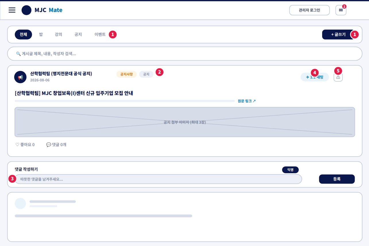
[SCR-07] 게시물 (커뮤니티) — 와이어프레임 (번호는 아래 구성요소 표와 대응)
