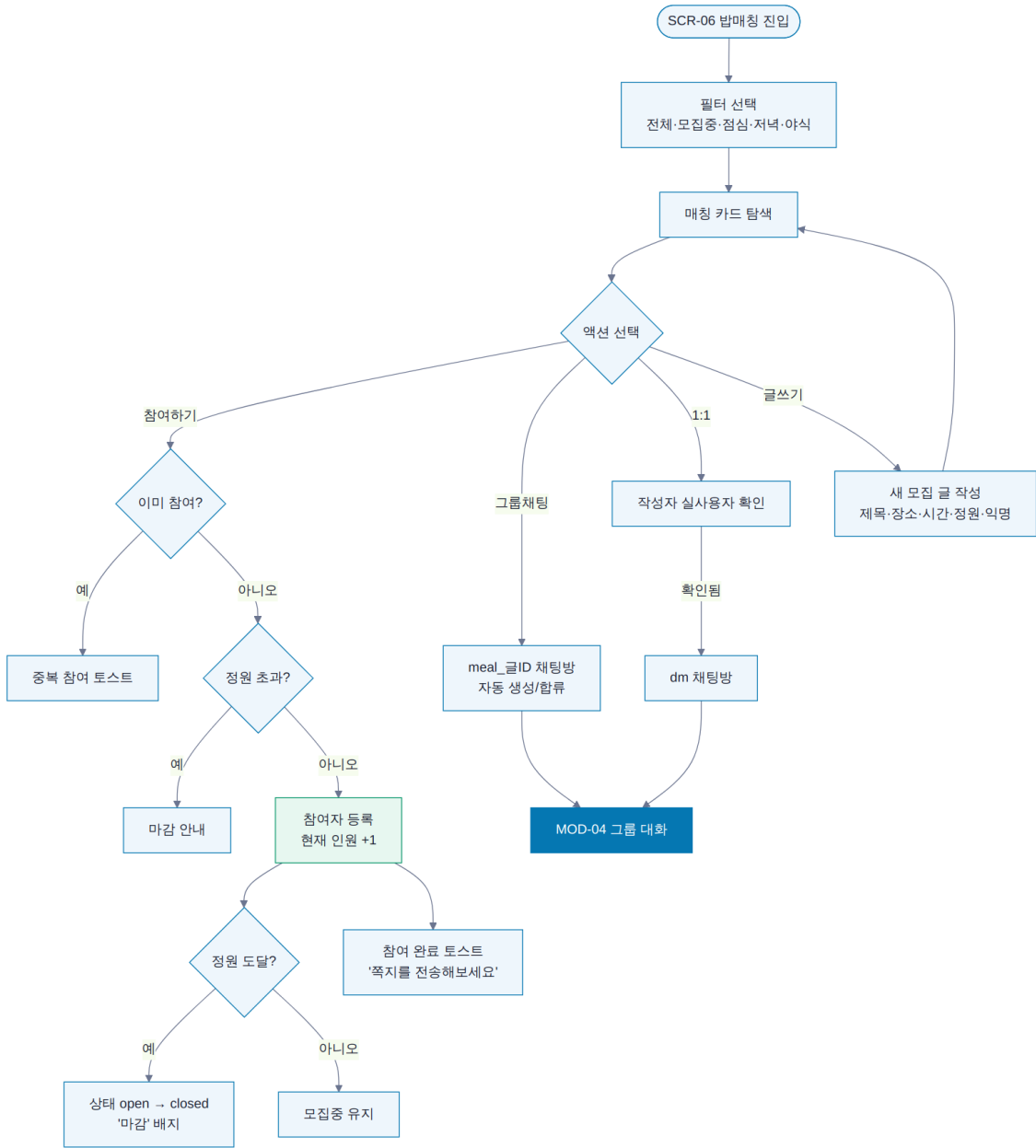
[UF-03] 밥매칭 참여 → 그룹채팅 플로우
