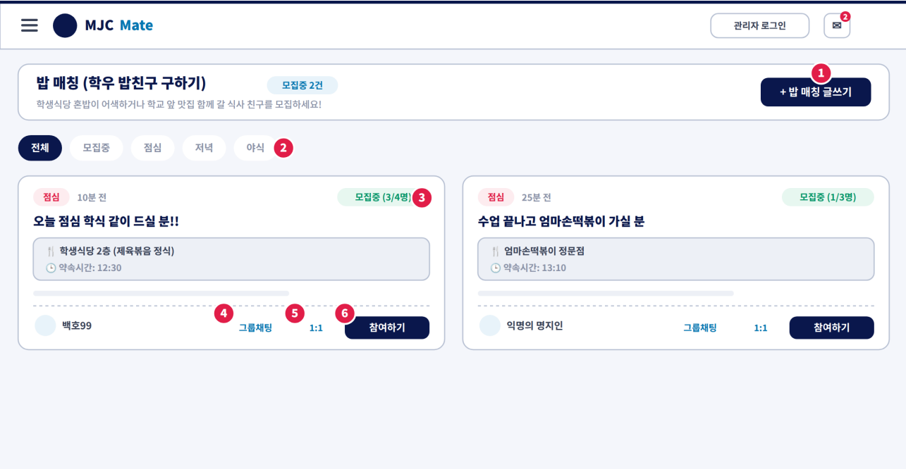
[SCR-06] 밥매칭 — 와이어프레임 (번호는 아래 구성요소 표와 대응)
