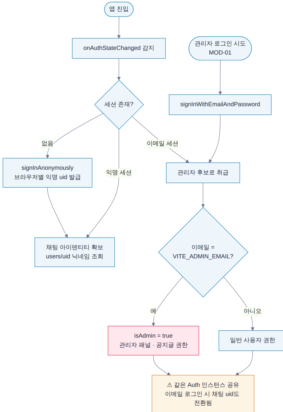
[SF-05] 인증 흐름 — 익명(채팅) vs 이메일(관리자)
