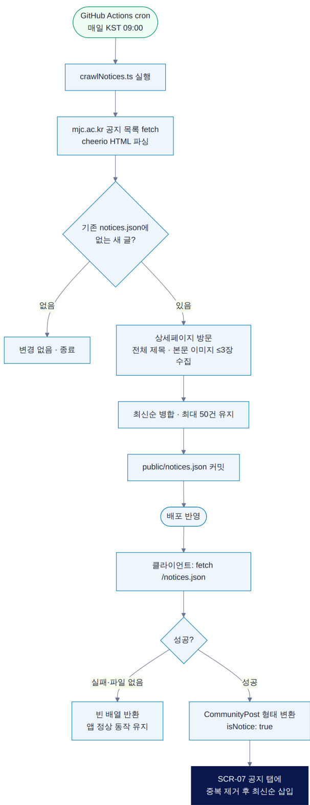
[SF-04] 학교 공지 크롤링 파이프라인
