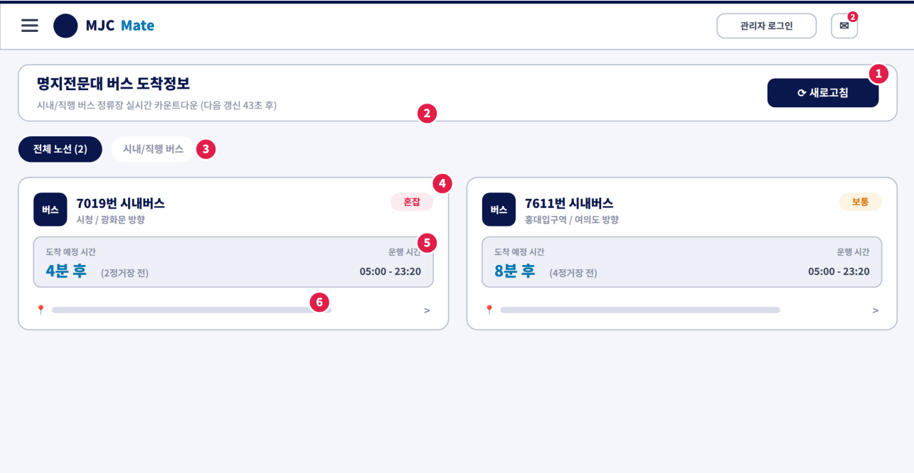
[SCR-02] 버스도착 — 와이어프레임 (번호는 아래 구성요소 표와 대응)
