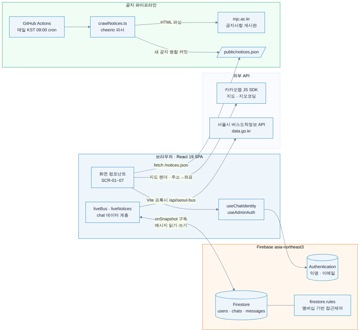
[SF-01] 전체 시스템 아키텍처
