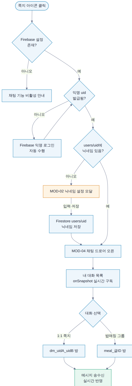
[UF-02] 실시간 채팅 최초 진입 플로우
