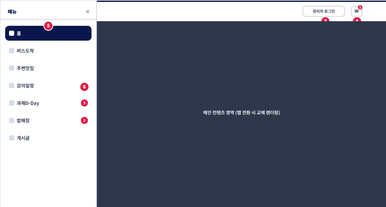
[CMN-01-02] 공통 레이아웃 — 헤더 & 사이드바 — 와이어프레임 (번호는 아래 구성요소 표와 대응)
