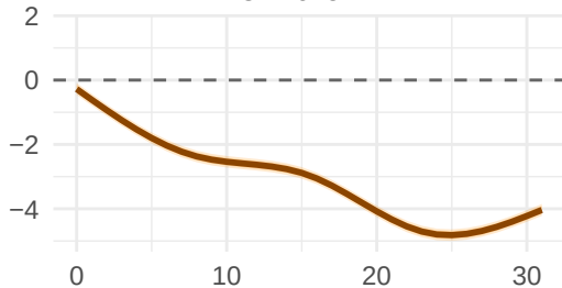
OLMo-3 7B
