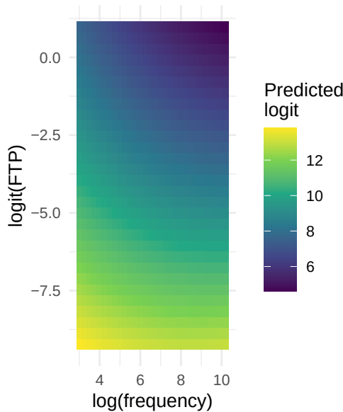
OLMo — final layer
