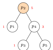
图注： p = [3, 1, 4, 2, 5] 的笛卡尔树；橙 = 根（全局最小）；红字 = 子树 size。答案 = 5! / (5 \cdot 1 \cdot 3 \cdot 1 \cdot 1) = 8 。
