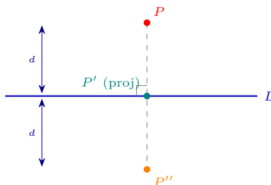
图注： P' （投影）是 P 到 L 的垂足； P'' （对称点）满足 P' 是 P, P'' 中点，从而 P'' = 2P' - P 。
