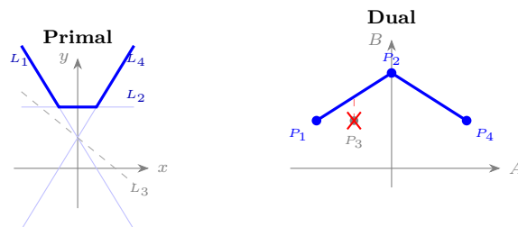
图注: 左 Primal 4 条线, 上半包络 = L_1 \rightarrow L_2 \rightarrow L_4 (粗蓝折线), L_3 全程在下被压 (灰虚线)。右 Dual 4 个对偶点, P_3 = (-1, 1) 严格落在弦 P_1P_2 下方 (红虚示意垂直差 0.5), 上凸壳 P_1 \rightarrow P_2 \rightarrow P_4 不收 P_3 。这就是「 L_i 可见 \iff P_i 在上凸壳上」的视觉对照。
