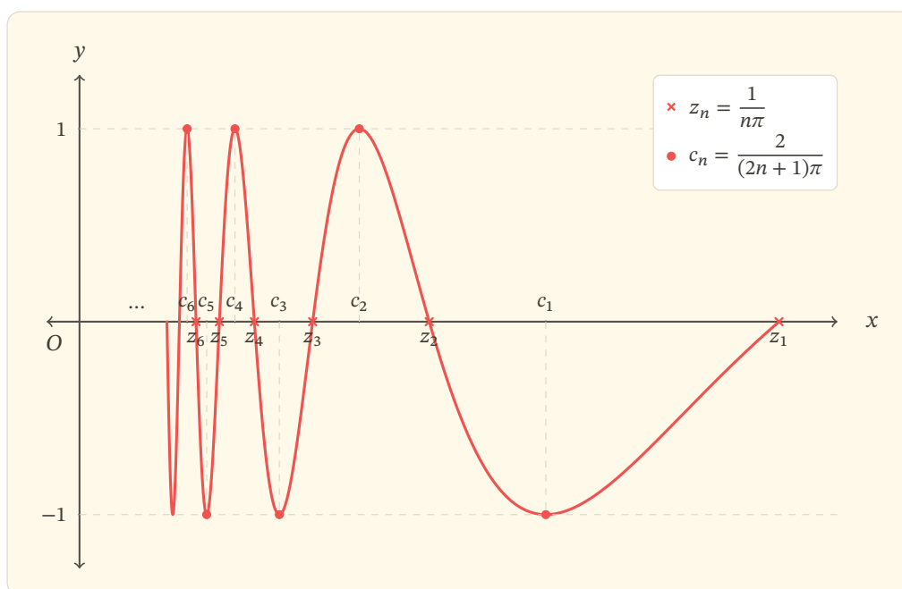
Hình 1: Các nghiệm z_n và hoành độ cực trị c_n xen kẽ, cùng dồn về 0 trên nửa trục dương.
