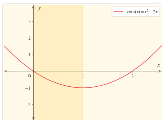
Đồ thị hàm số
