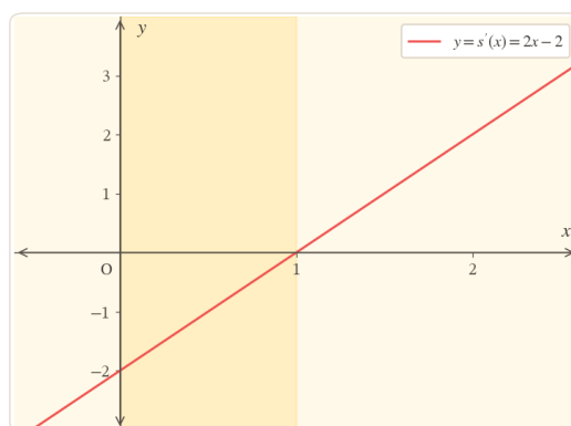
Đồ thị đạo hàm
