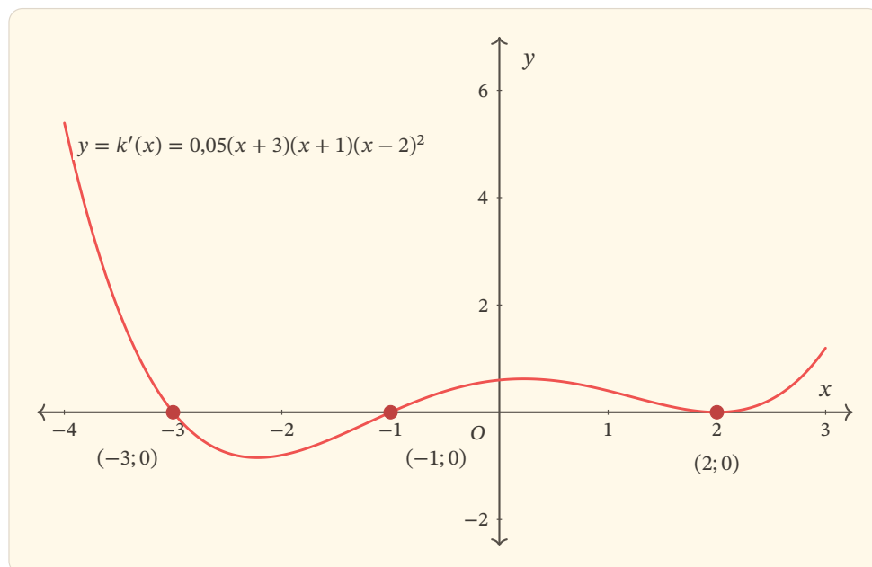
Bài kiểm tra 02 — Đồ thị đạo hàm trên khoảng (-4; 3) .
