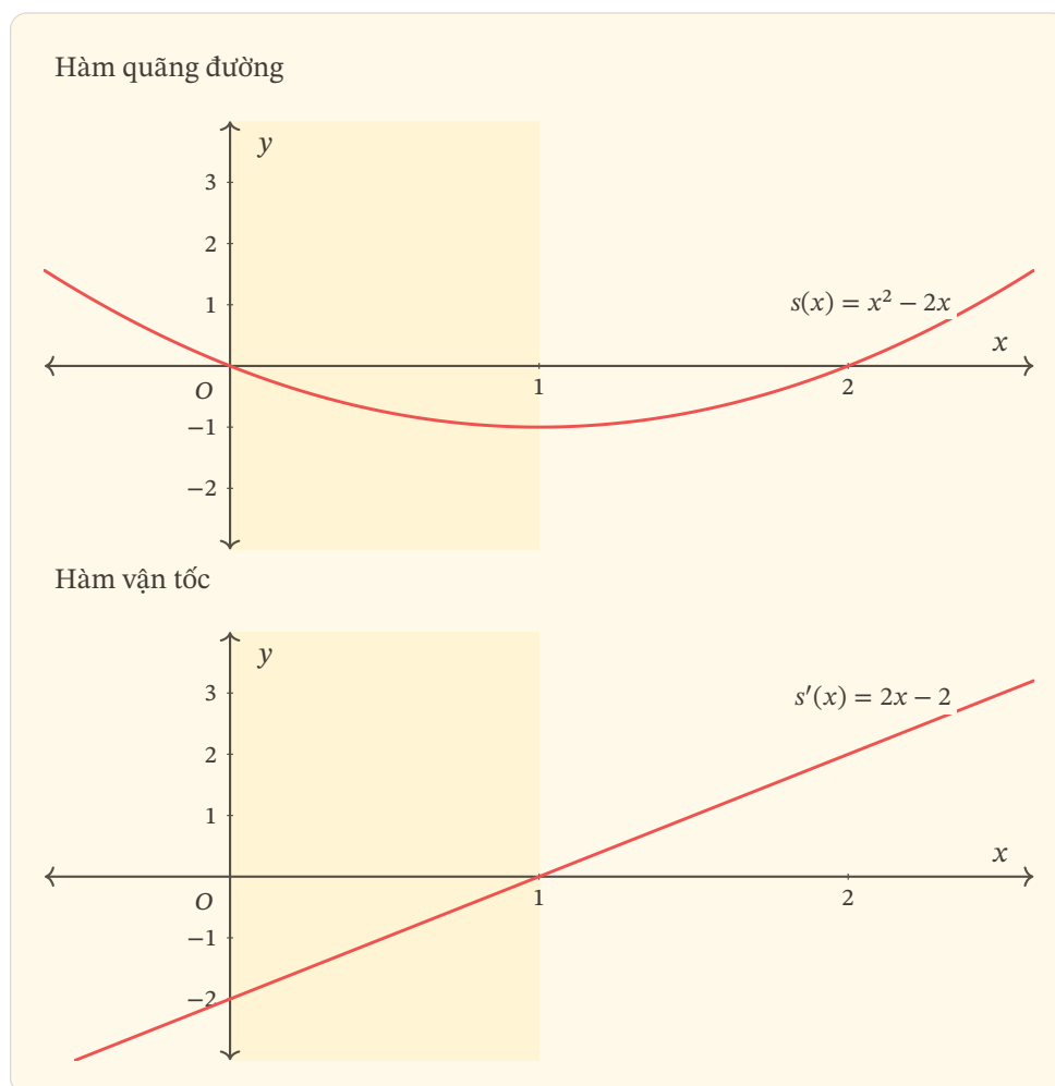
Hình 04 — Hai nhận khác nhau: s đang giảm trong khi s' đang tăng và mang giá trị âm trên (0; 1) .
