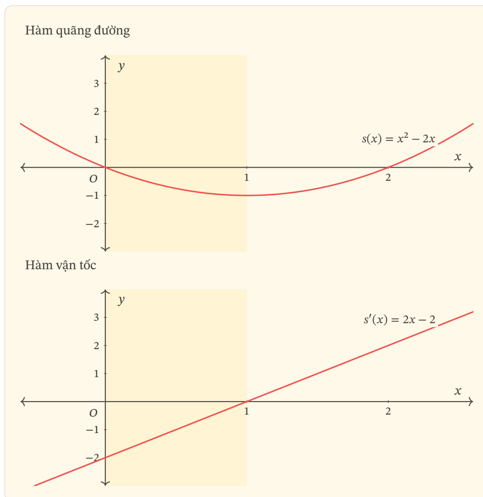
Hình 04 — Hai nhần khác nhau: s đang giảm trong khi s' đang tăng và mang giá trị âm trên (0; 1) .
