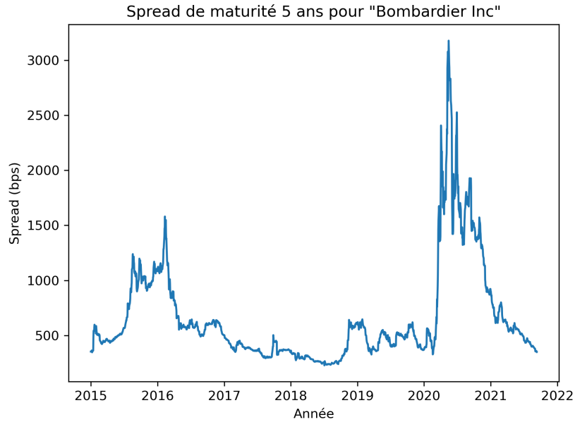
FIGURE 8.3 – Spread de maturité 5 ans pour Bombardier Inc
