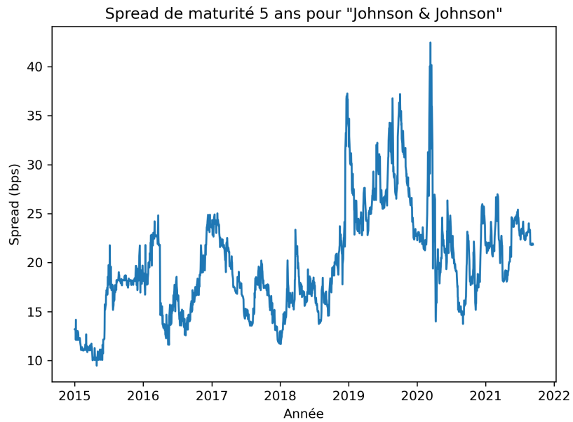
FIGURE 8.1 – Spread de maturité 5 ans pour Johnson & Johnson
