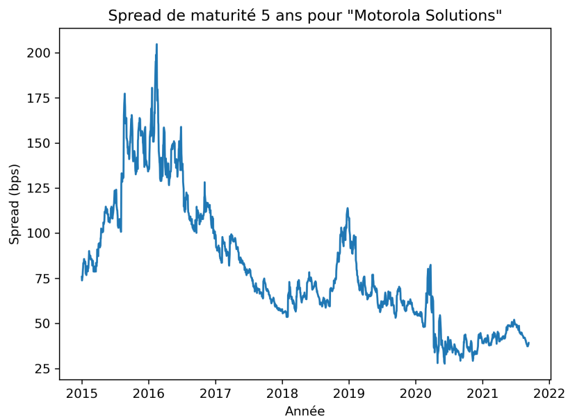
FIGURE 8.2 – Spread de maturité 5 ans pour Motorola Solutions
