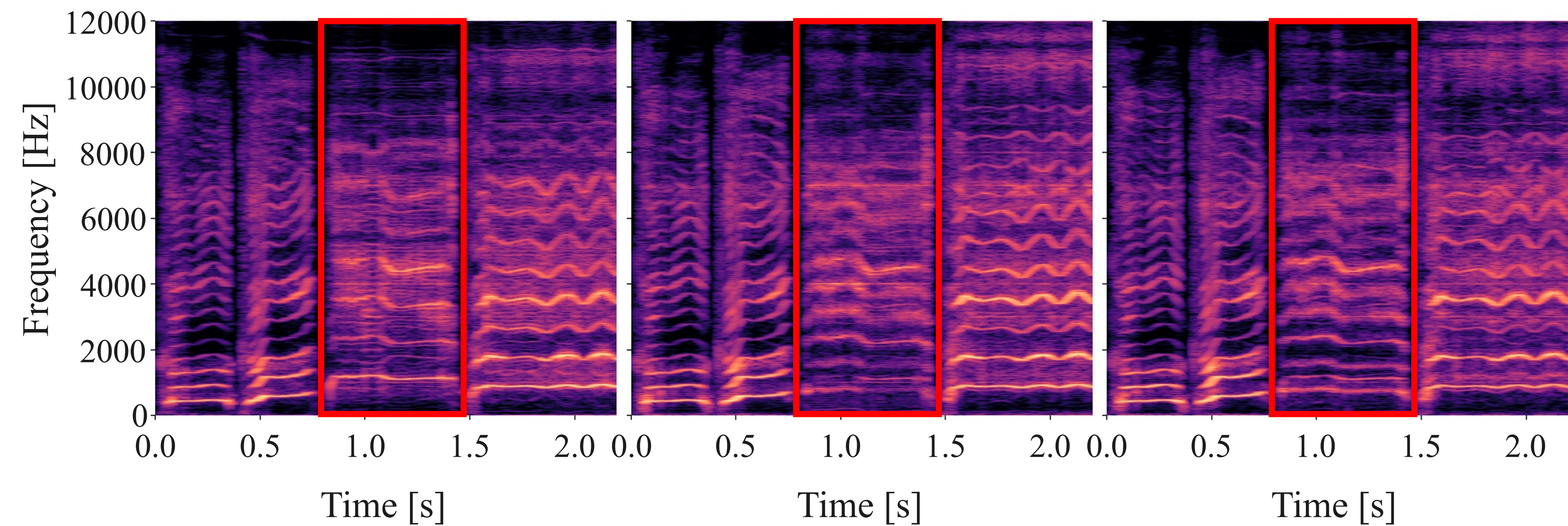
(a) SiFi-GAN
