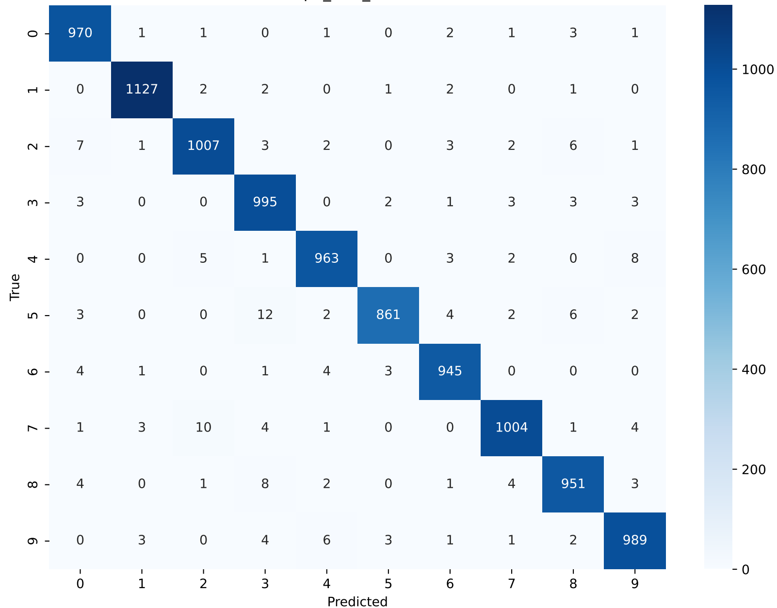
exp1_MLP_Shallow
