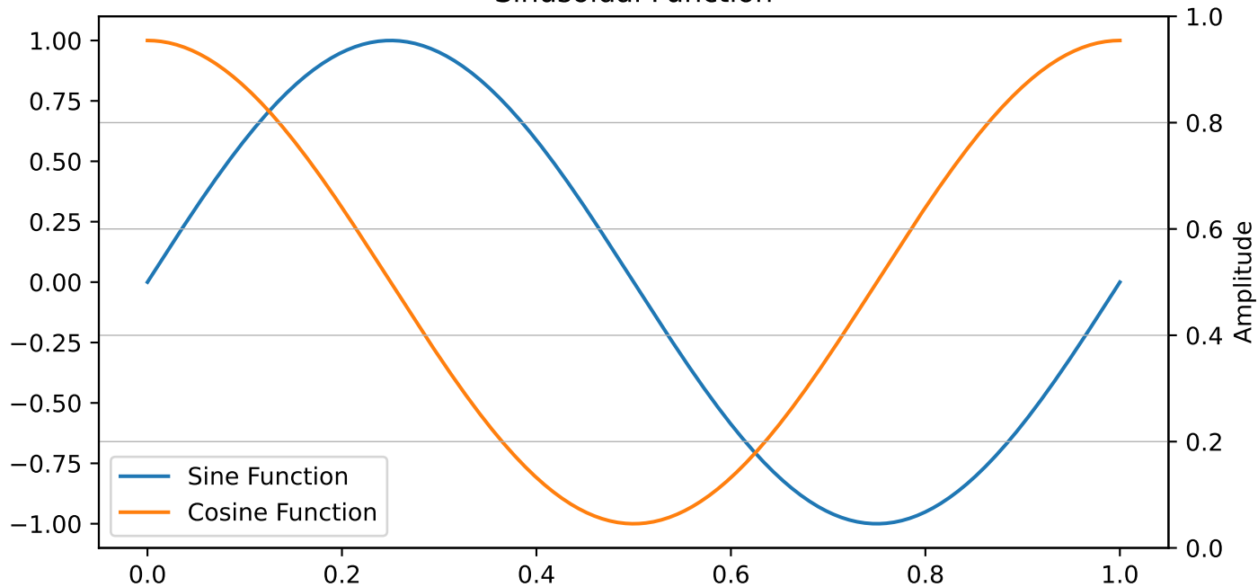
Sinusoidal Function
