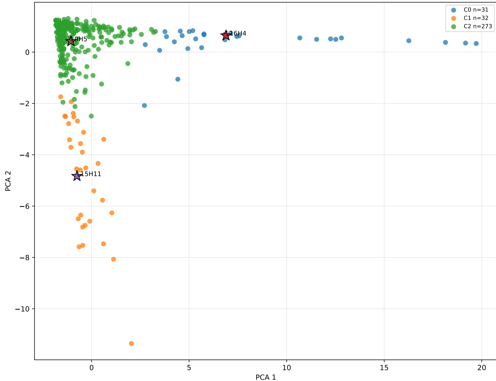
ctx_0088_answer_to_rag_x_cluster PCA
