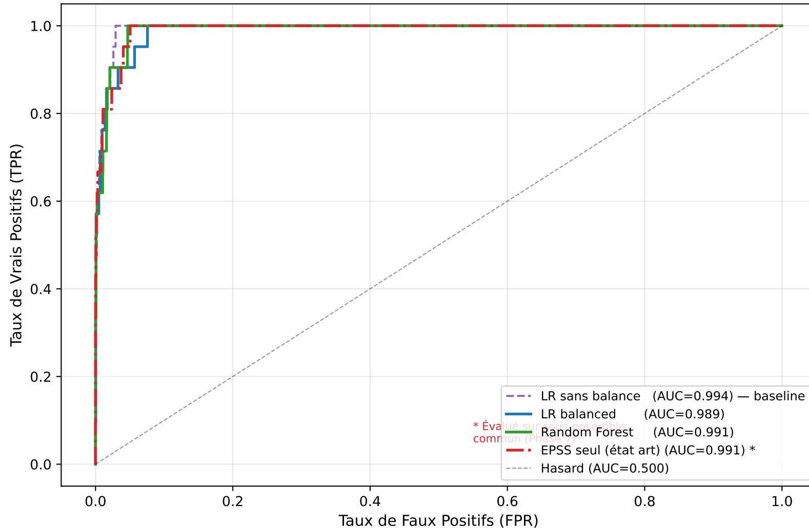
Courbes ROC — Paradigme 2 : CVSS + EPSS (7 CWE Auth/Authz — CISA KEV comme vérité terrain)
