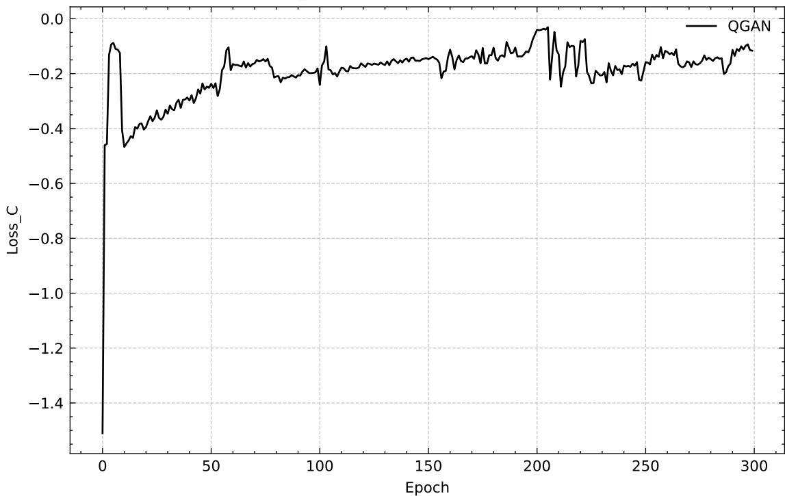
So sánh Loss_C theo Epoch (không bao gồm W-GAN)
