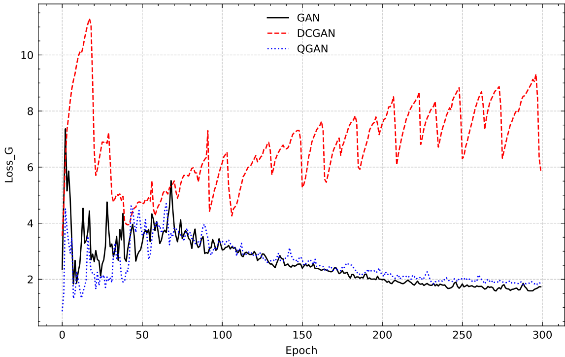
So sánh Loss_G (không bao gồm WGAN)
