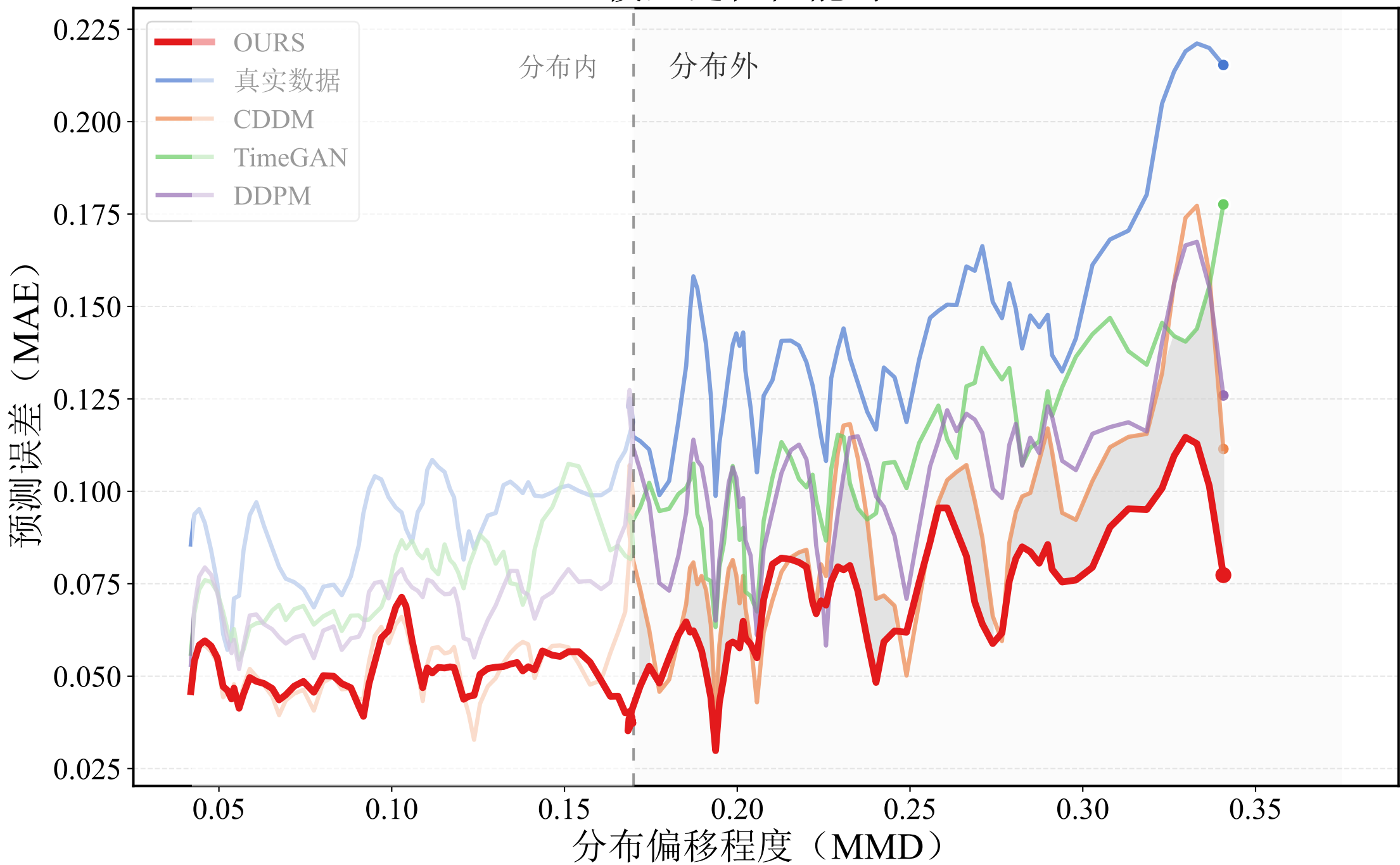
模型泛化性能对比
