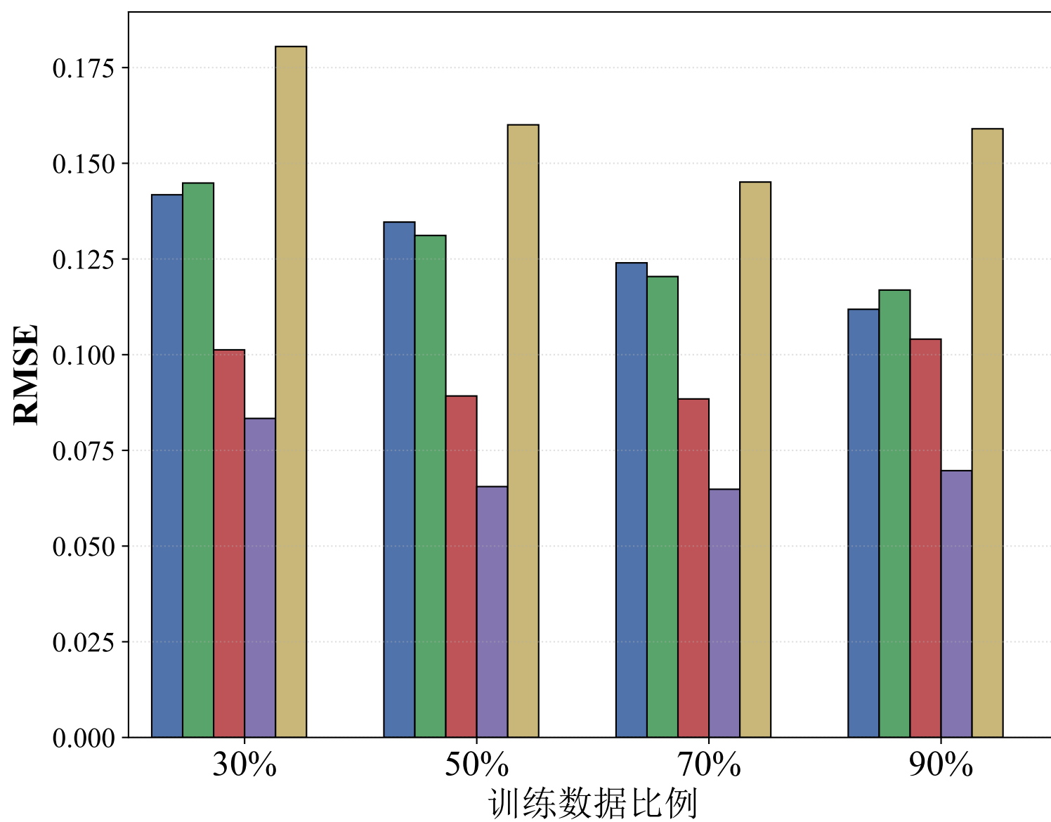
(c) RMSE 对比结果
