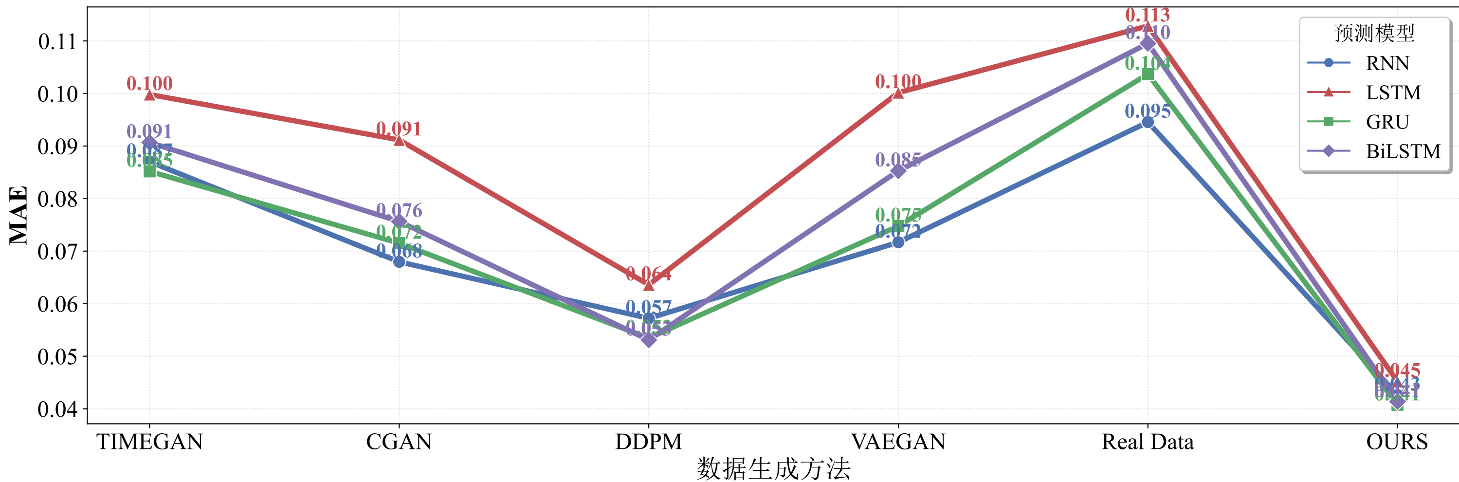
不同预测模型在 70% 训练数据条件下的 MAE 对比
