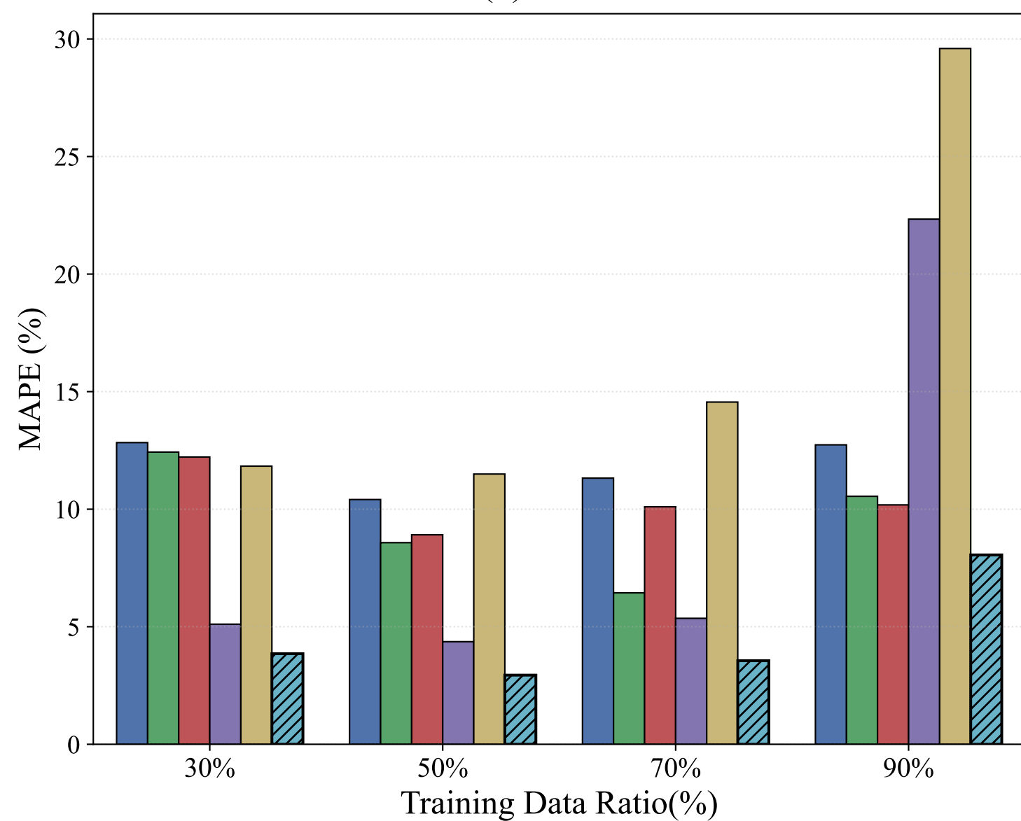
(d) MAPE
