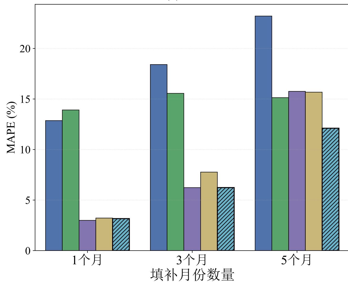
(d) MAPE
