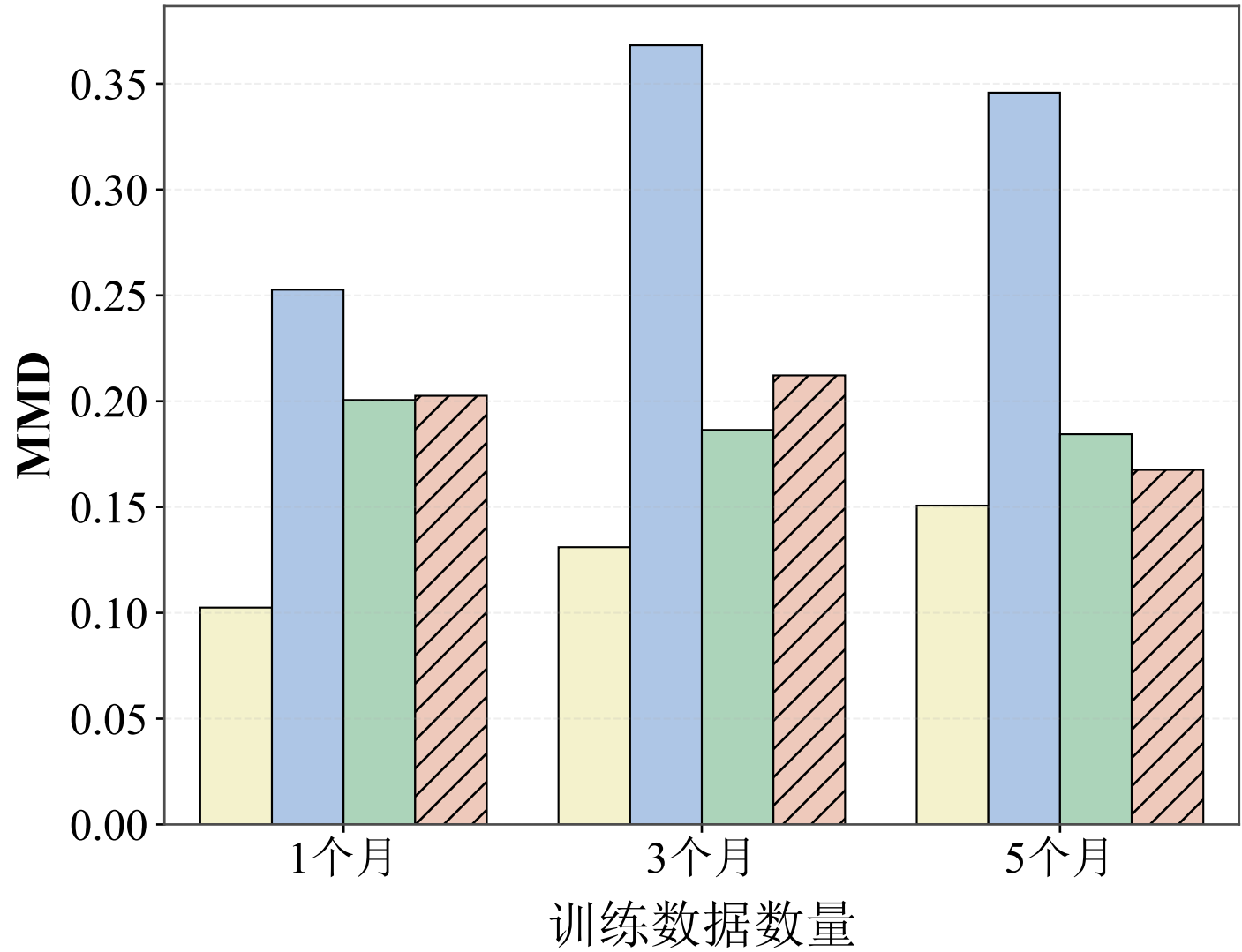
与训练数据的分布差异(MMD)
