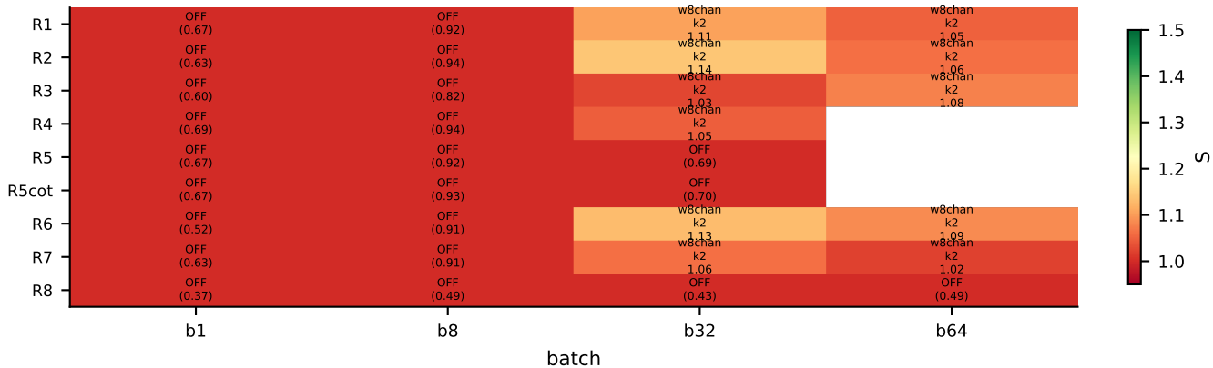
mla: real-data winner per dataset x batch (Stage B; S vs AR)
